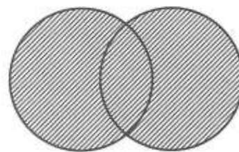
図2. OR 検索
