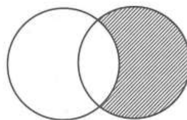
図3. NOT 検索
